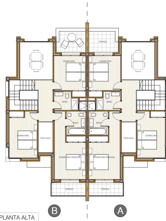
PLANTA ALTA
