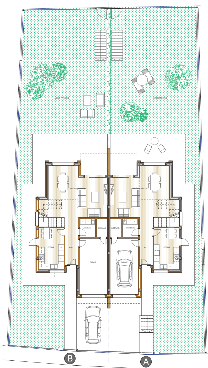
PLANTA BAJA
